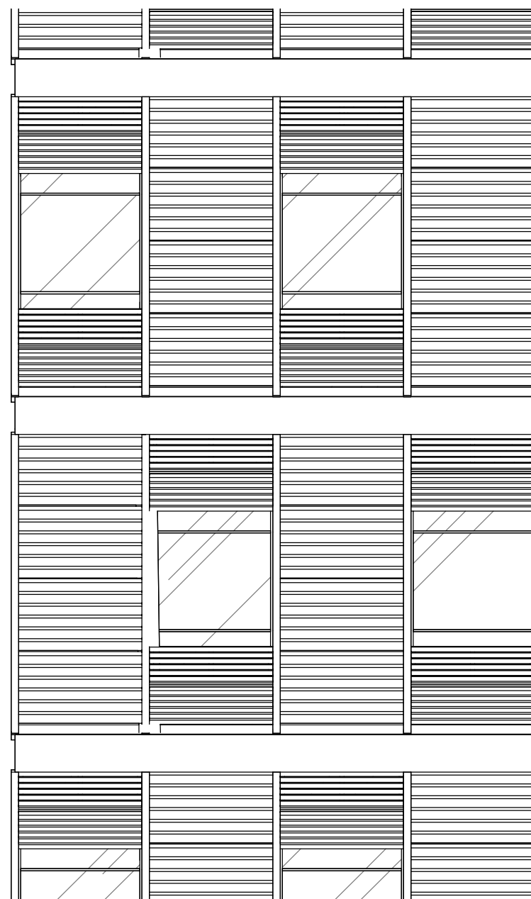
2 ELEVAÇÃO 1 : 50
