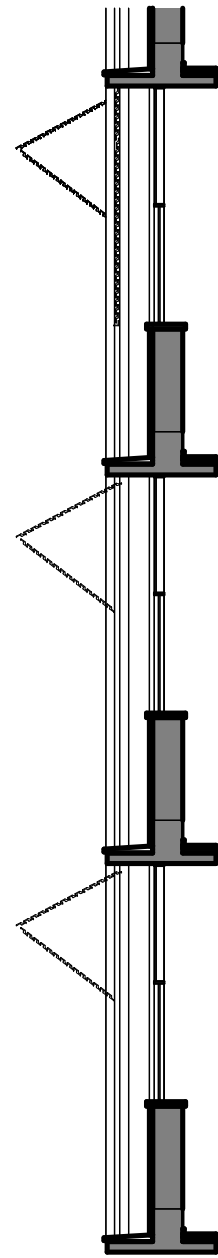
1 CORTE 1 : 50
