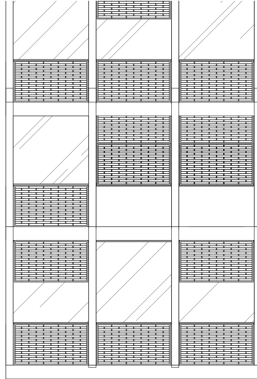
2 ELEVAÇÃO 1 : 50
