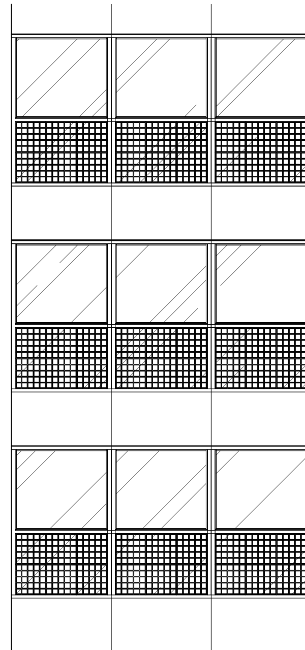
2 ELEVAÇÃO 1 : 50
