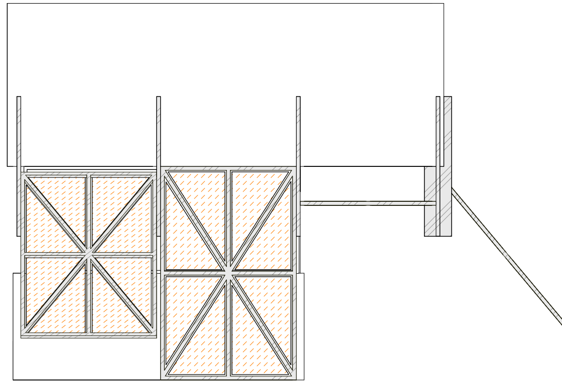
ELEVAÇÃO ESC: 1 : 50
