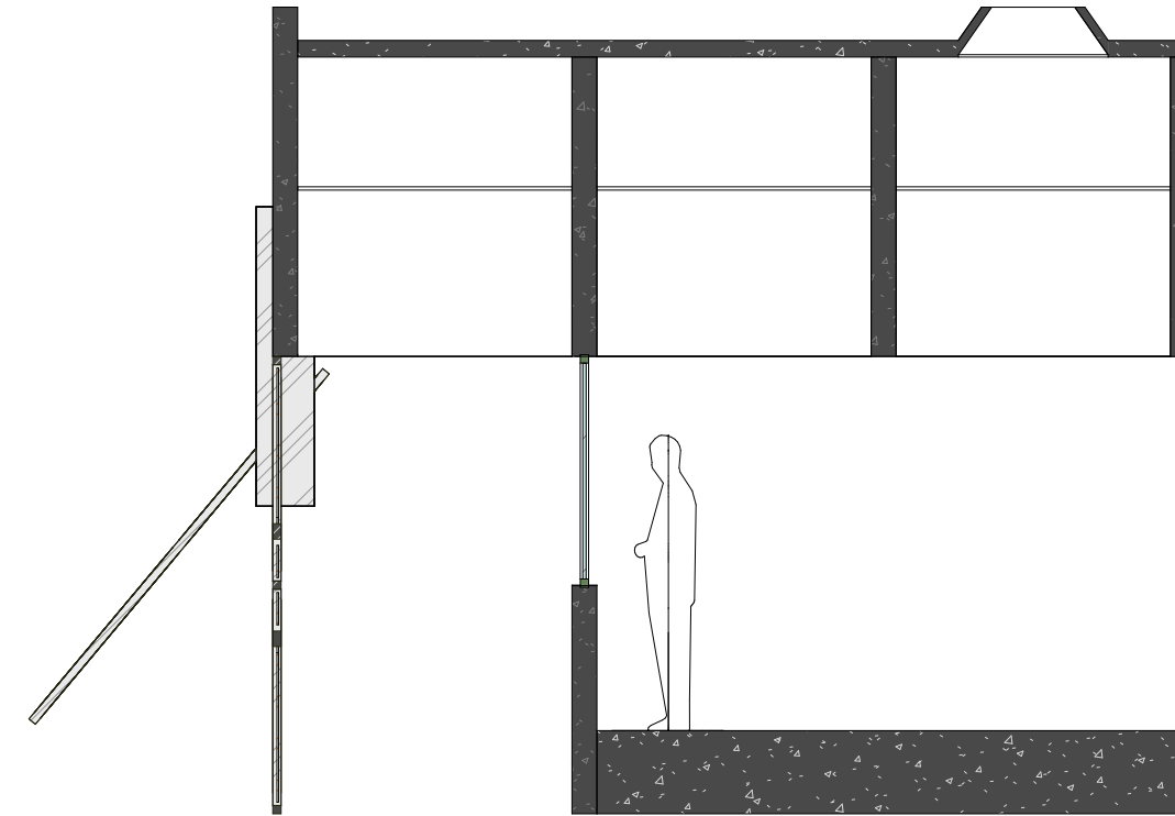
CORTE A ESC: 1 : 50
